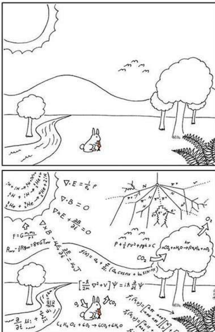
Figura 1: Algunos cambios infinitesimales en un sistema.
